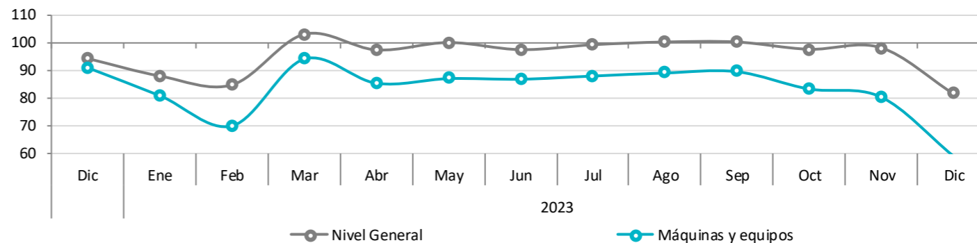
Gráfico 22. ISIM-PBA Nivel general y bloque Máquinas y equipos (*) (**). Período diciembre 2022 - diciembre 2023. Índice base 2012=100
