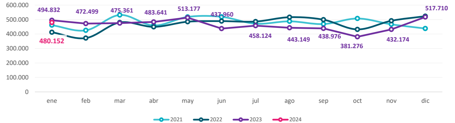
Gráfico 49. Provincia de Buenos Aires. Producción de gasoil común Período enero 2021 – enero 2024. En metros cúbicos
