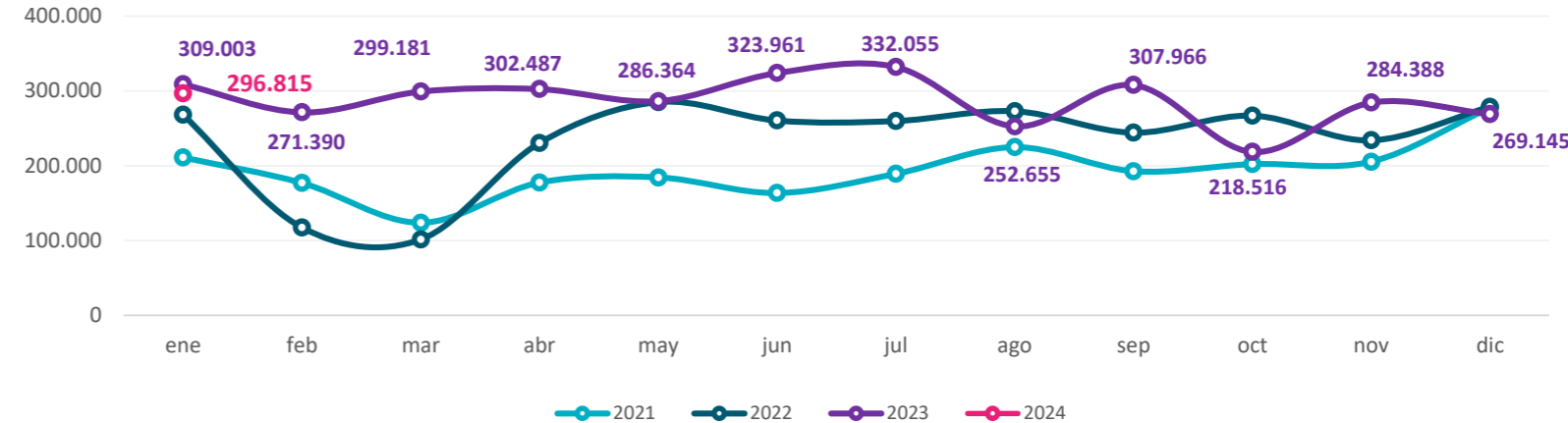
Gráfico 51. Provincia de Buenos Aires. Producción de gasoil ultra Período enero 2021 – enero 2024. En metros cúbicos
