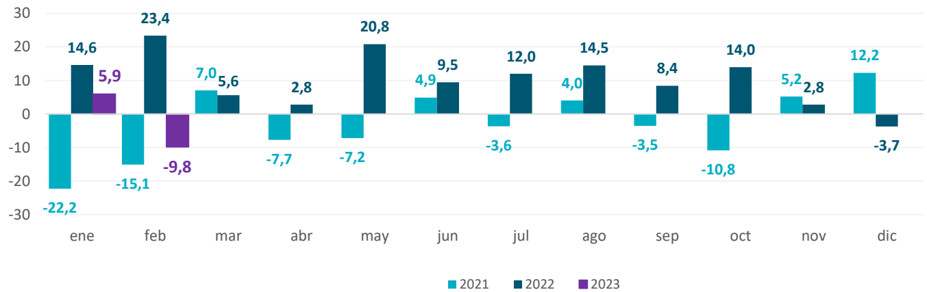
Gráfico 30. Provincia de Buenos Aires. Faena avícola Período enero 2021 – febrero 2023. Variación porcentual interanual
