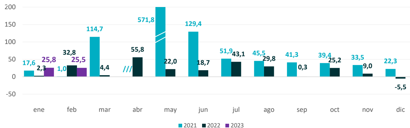
Gráfico 42. Provincia de Buenos Aires. Producción de vehículos Período enero 2021 – febrero 2023. Variación porcentual interanual
