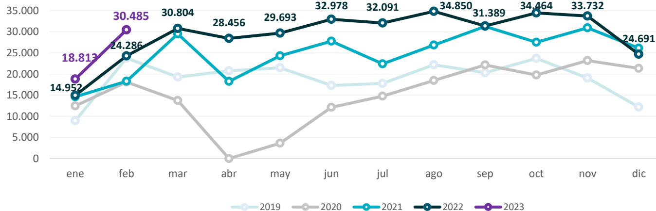
Gráfico 41. Provincia de Buenos Aires. Producción de vehículos Período enero 2019 – febrero 2023. En unidades
