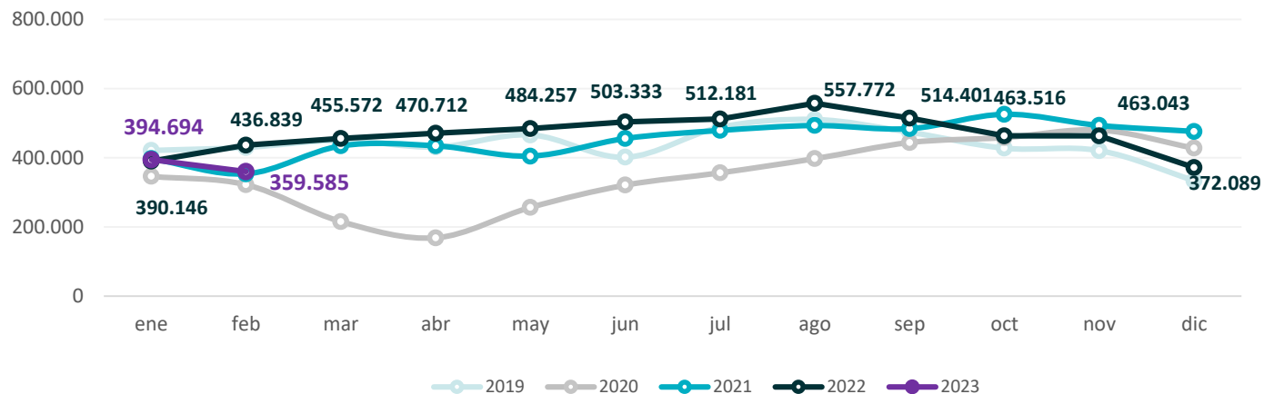
Gráfico 39. Provincia de Buenos Aires. Despacho de cemento Período enero 2019 – febrero 2023. En toneladas
