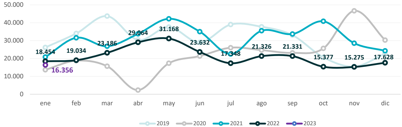
Gráfico 57. Provincia de Buenos Aires. Producción de asfalto Período enero 2019 – enero 2023. En metros cúbicos
