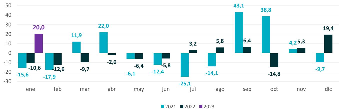
Gráfico 50. Provincia de Buenos Aires. Producción de gasoil común Período enero 2021 – enero 2023. Variación porcentual interanual
