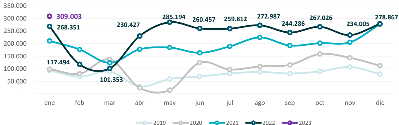
Gráfico 51. Provincia de Buenos Aires. Producción de gasoil ultra Período enero 2019 – enero 2023. En metros cúbicos
