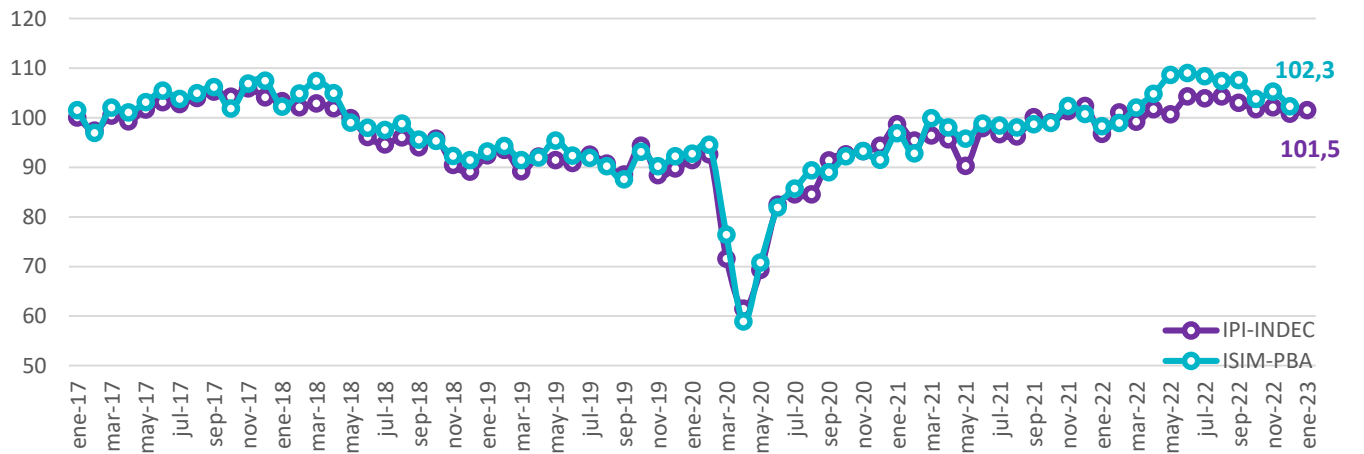
Gráfico 4. IPI-INDEC e ISIM-PBA (*) (**). Serie desestacionalizada Período enero 2017 – enero 2023. Índice Base 2016 = 100
