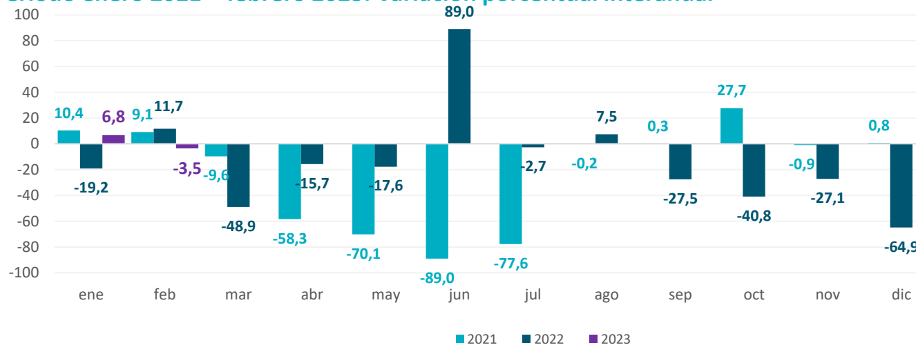
Gráfico 22. Provincia de Buenos Aires. Pellets de soja Período enero 2021 – febrero 2023. Variación porcentual interanual
