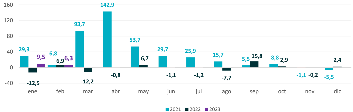
Gráfico 38. Provincia de Buenos Aires. Producción de cemento Período enero 2021 – febrero 2023. Variación porcentual interanual
