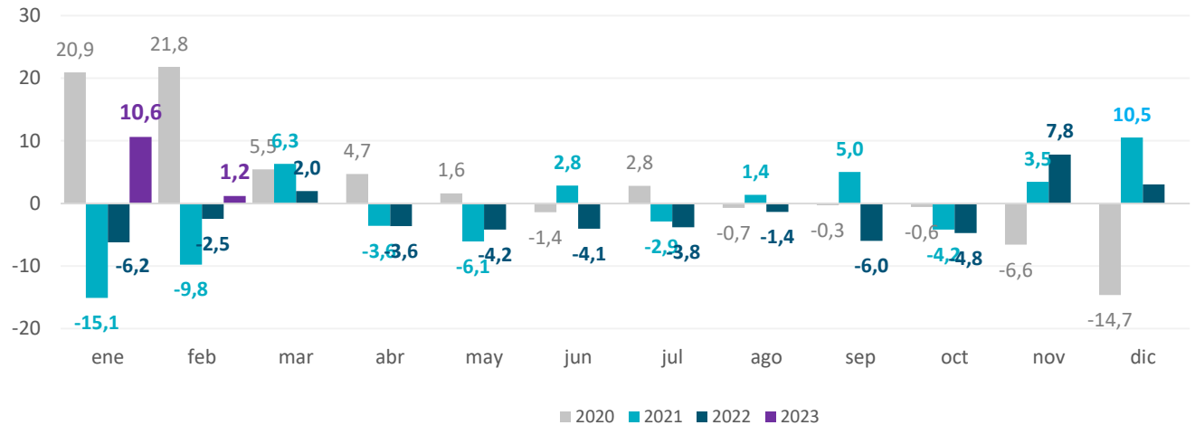
Gráfico 8. Provincia de Buenos Aires. Molienda de trigo pan Período enero 2021 – febrero 2023. Variación porcentual interanual
