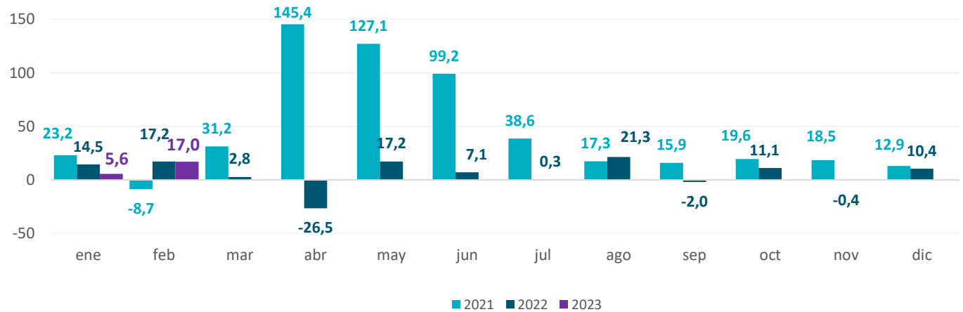
Gráfico 36. Provincia de Buenos Aires. Producción de acero crudo Período enero 2021 – febrero 2023. Variación porcentual interanual
