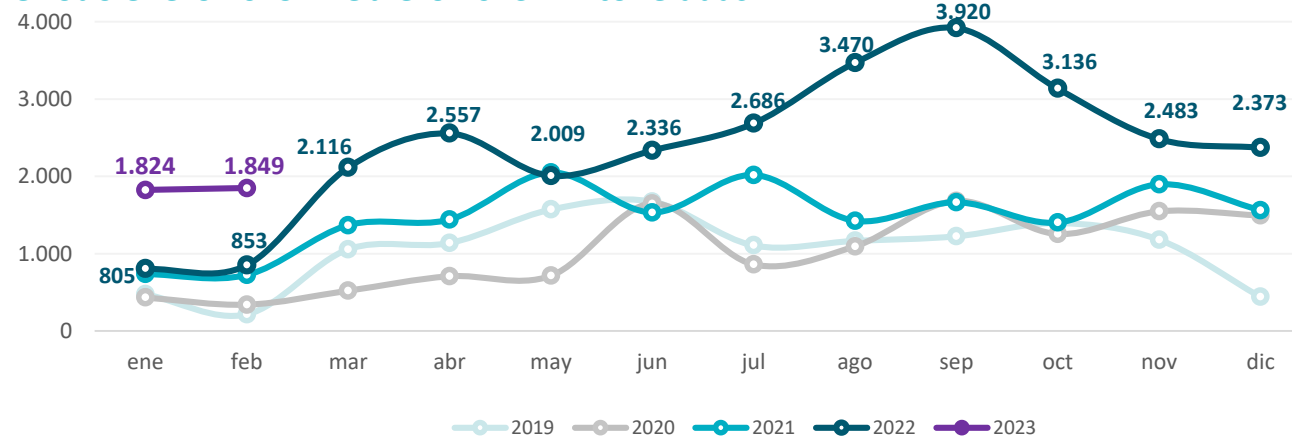
Gráfico 19. Provincia de Buenos Aires. Expellers de girasol Período enero 2019 – febrero 2023. En toneladas
