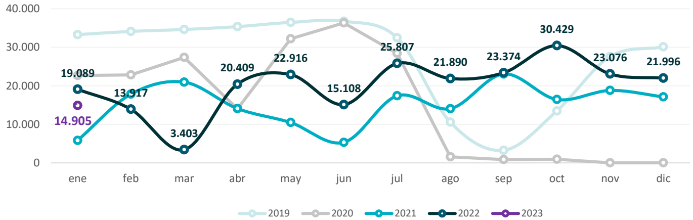
Gráfico 58. Provincia de Buenos Aires. Producción de biodiesel Período enero 2019 – enero 2023. En toneladas
