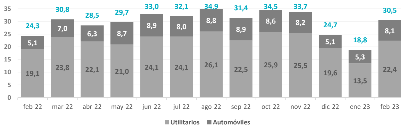
Gráfico 43. Provincia de Buenos Aires. Producción de vehículos por categoría Período febrero 2022– febrero 2023. En miles de unidades
