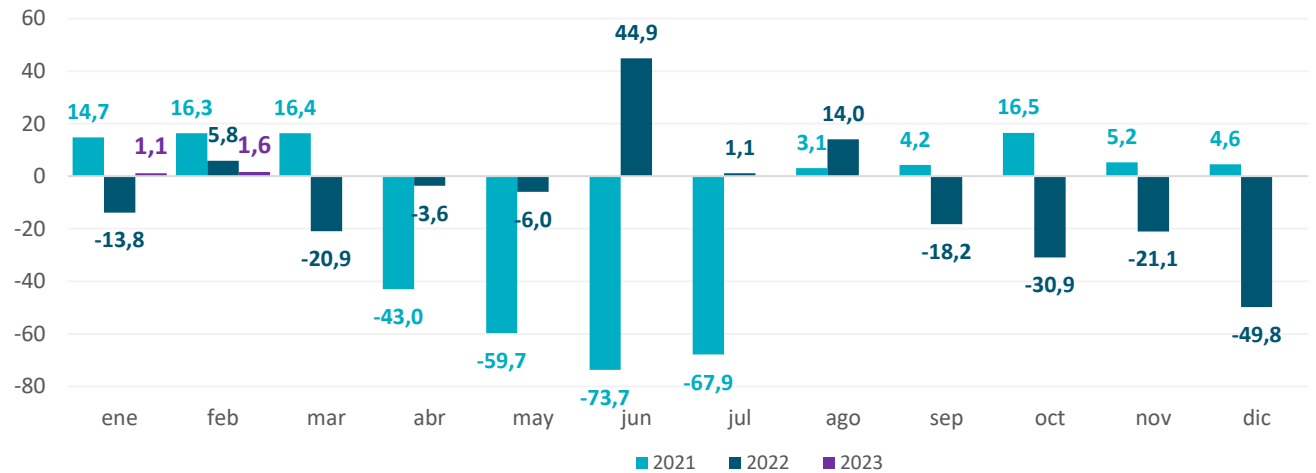
Gráfico 10. Provincia de Buenos Aires. Molienda de soja Período enero 2021 – febrero 2023. Variación porcentual interanual
