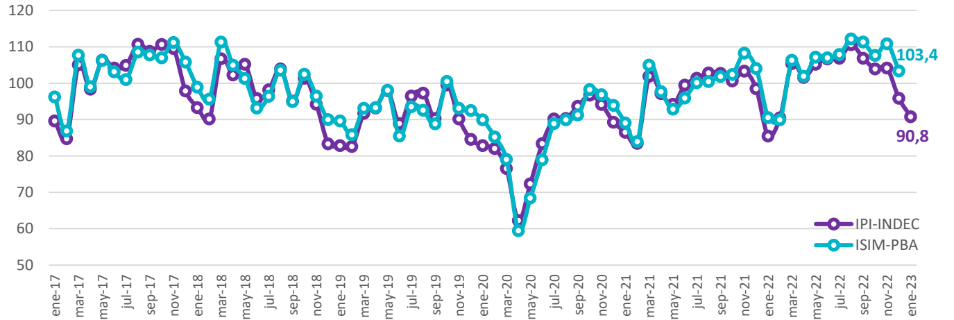
Gráfico 3. IPI-INDEC e ISIM-PBA (*) (**). Nivel general Período enero 2017 – enero 2023. Índice Base 2016 = 100
