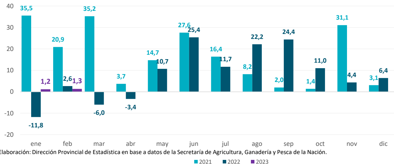
Gráfico 18. Provincia de Buenos Aires. Expellers de soja Período enero 2021 – febrero 2023. Variación porcentual interanual
