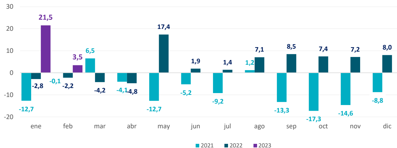
Gráfico 26. Provincia de Buenos Aires. Faena bovina Período enero 2021 – febrero 2023. Variación porcentual interanual
