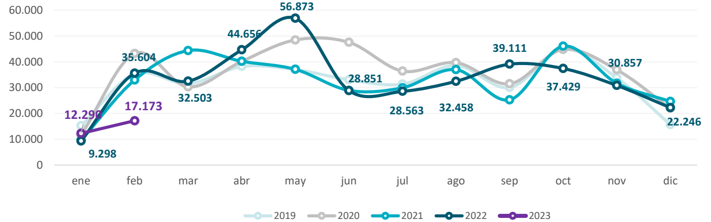
Gráfico 31. Provincia de Buenos Aires. Desembarques de capturas pesqueras Período enero 2019 – febrero 2023. En toneladas
