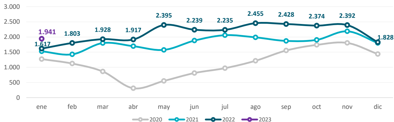
Gráfico 5. Provincia de Buenos Aires. Producción transportada de minerales. Período enero 2020 – enero 2023. En miles de toneladas
