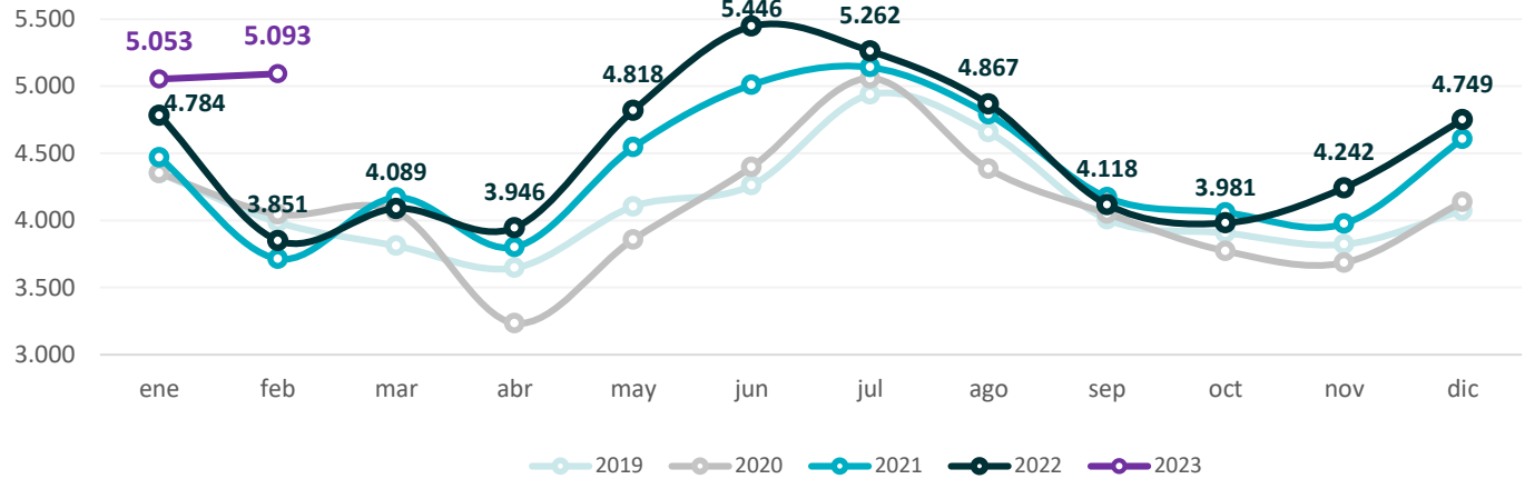
Gráfico 62. Provincia de Buenos Aires. Demanda eléctrica Período enero 2019 – febrero 2023. En Gwh
