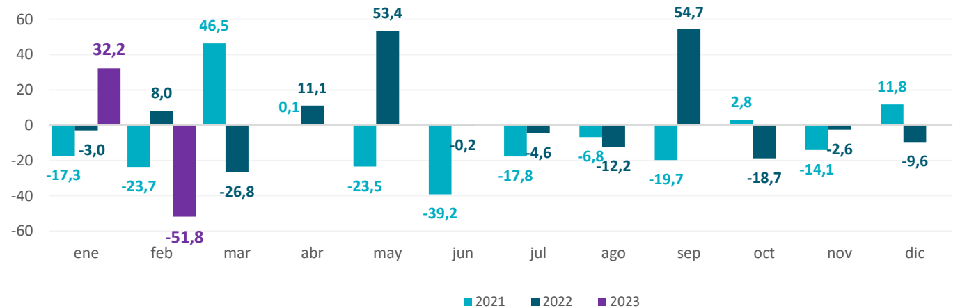
Gráfico 32. Provincia de Buenos Aires. Desembarques de capturas pesqueras Período enero 2021 – febrero 2023. Variación porcentual interanual
