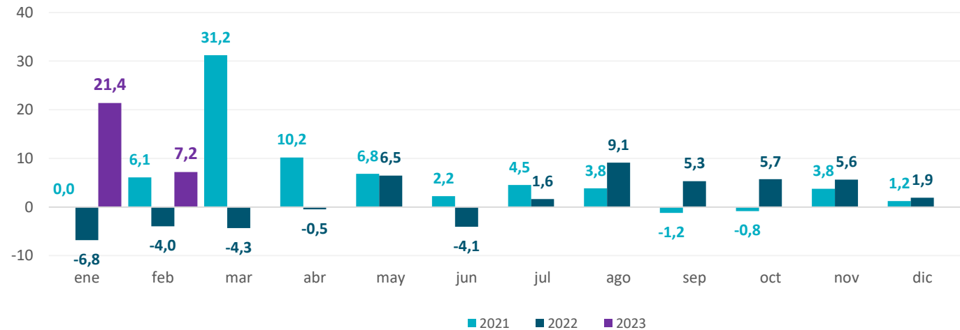
Gráfico 28. Provincia de Buenos Aires. Faena porcina Período enero 2021 – febrero 2023. Variación porcentual interanual
