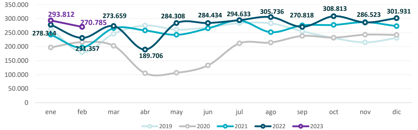
Gráfico 35. Provincia de Buenos Aires. Producción de acero crudo Período enero 2019 – febrero 2023. En toneladas
