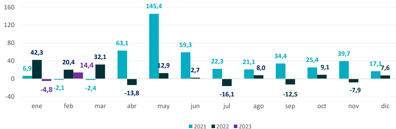
Gráfico 34. Provincia de Buenos Aires. Producción de hierro primario Período enero 2021 – febrero 2023. Variación porcentual interanual
