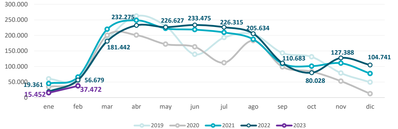
Gráfico 11. Provincia de Buenos Aires. Molienda de girasol Período enero 2019 – febrero 2023. En toneladas
