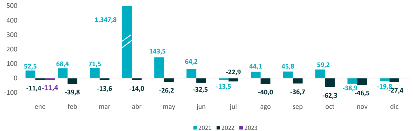
Gráfico 58. Provincia de Buenos Aires. Producción de asfalto Período enero 2021 – enero 2023. Variación porcentual interanual
