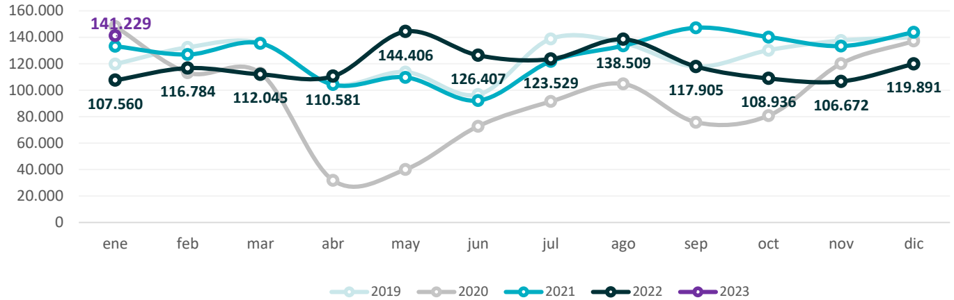
Gráfico 55. Provincia de Buenos Aires. Producción de nafta ultra Período enero 2019 – enero 2023. En metros cúbicos
