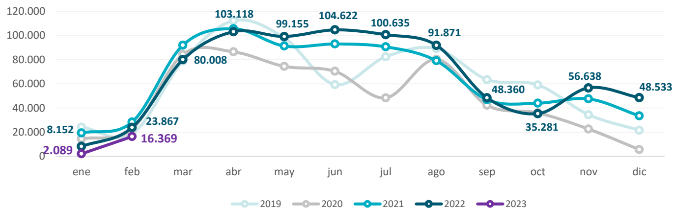
Gráfico 15. Provincia de Buenos Aires. Aceite de girasol Período enero 2019 – febrero 2023. En toneladas
