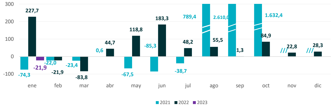
Gráfico 59. Provincia de Buenos Aires. Producción de biodiesel Período enero 2021 – enero 2023. Variación porcentual interanual
