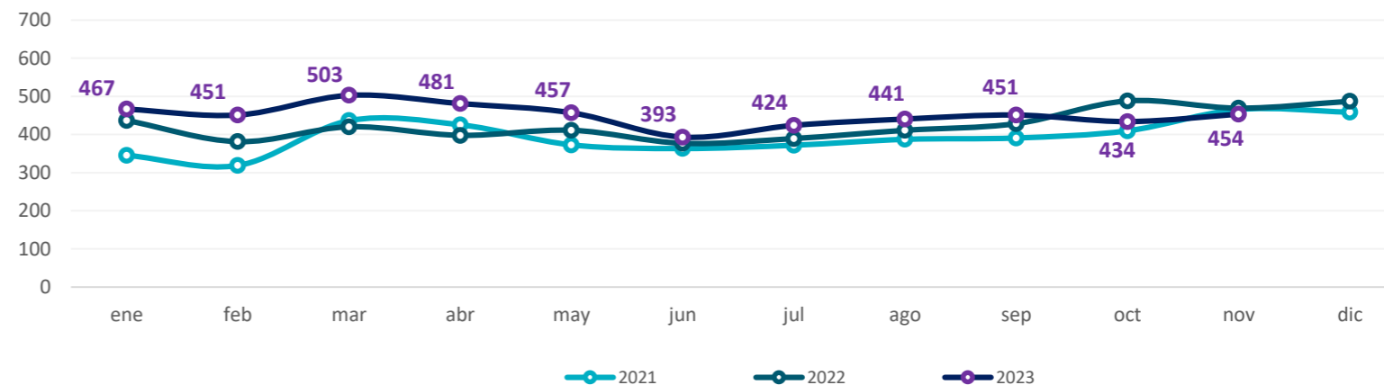
Gráfico 64. Provincia de Buenos Aires. Gas entregado a usuarios industriales Período enero 2021 – noviembre 2023. En millones de m 3 de 9.300 kcal
