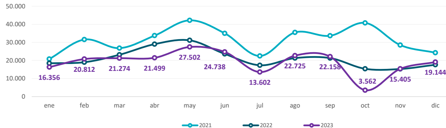
Gráfico 57. Provincia de Buenos Aires. Producción de asfalto Período enero 2021 – diciembre 2023. En metros cúbicos
