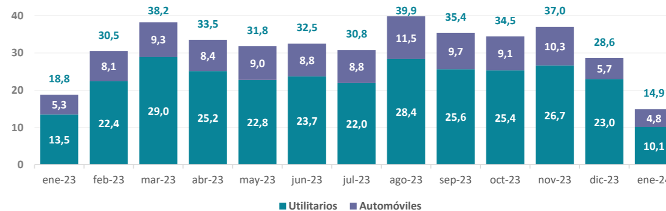
Gráfico 43. Provincia de Buenos Aires. Producción de vehículos por categoría Período enero 2023 – enero 2024. En miles de unidades
