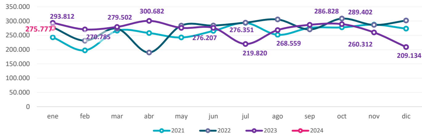
Gráfico 35. Provincia de Buenos Aires. Producción de acero crudo Período enero 2021 – enero 2024. En toneladas
