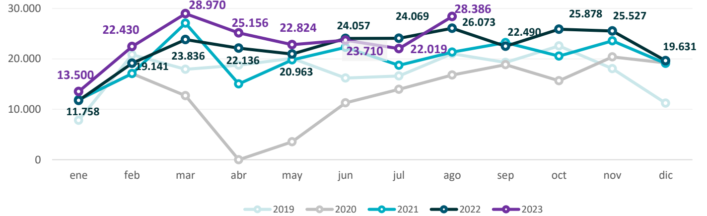
Gráfico 45. Provincia de Buenos Aires. Producción de vehículos utilitarios Período enero 2019 – agosto 2023. En unidades
