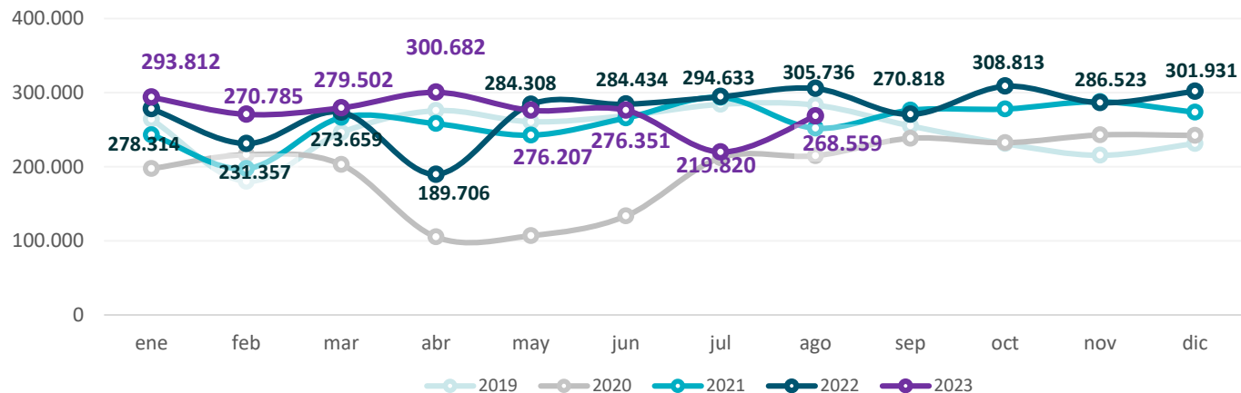
Gráfico 35. Provincia de Buenos Aires. Producción de acero crudo Período enero 2019 – agosto 2023. En toneladas
