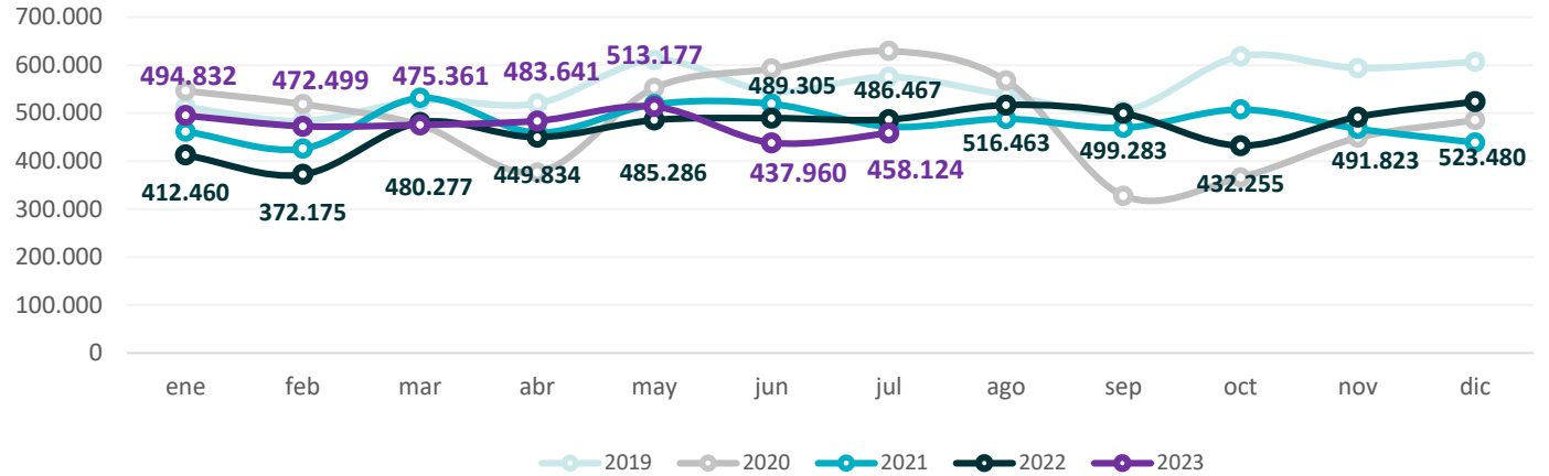
Gráfico 49. Provincia de Buenos Aires. Producción de gasoil común Período enero 2019 – julio 2023. En metros cúbicos
