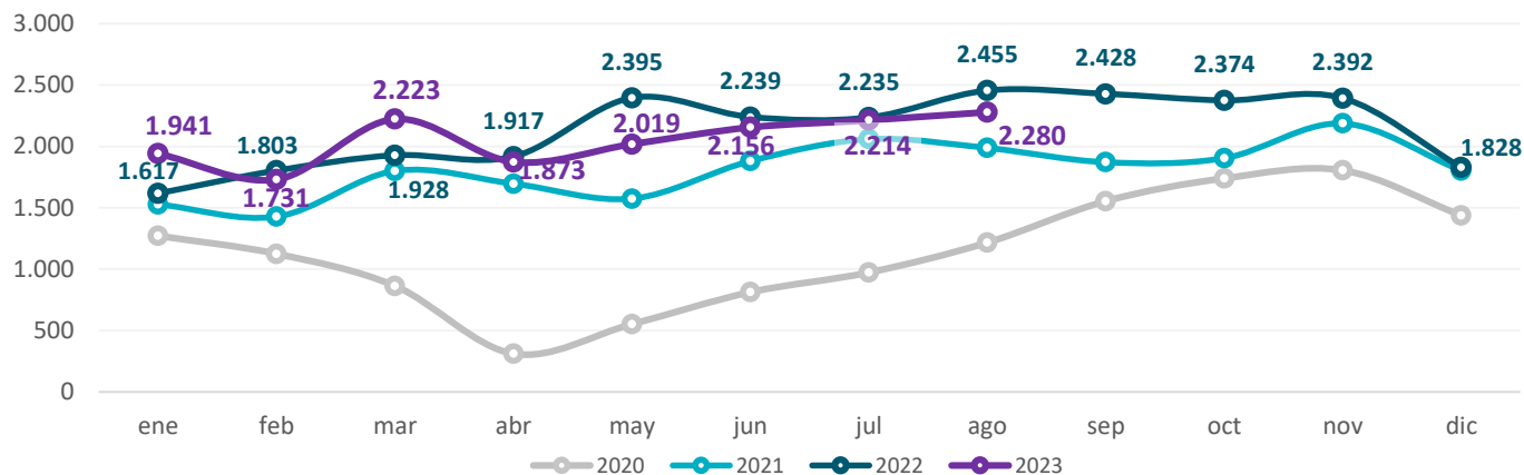
Gráfico 5. Provincia de Buenos Aires. Producción transportada de minerales. Período enero 2020 – agosto 2023. En miles de toneladas
