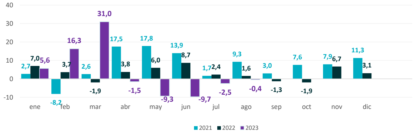
Gráfico 63. Provincia de Buenos Aires. Demanda eléctrica Período enero 2020 – agosto 2023. Variación porcentual interanual
