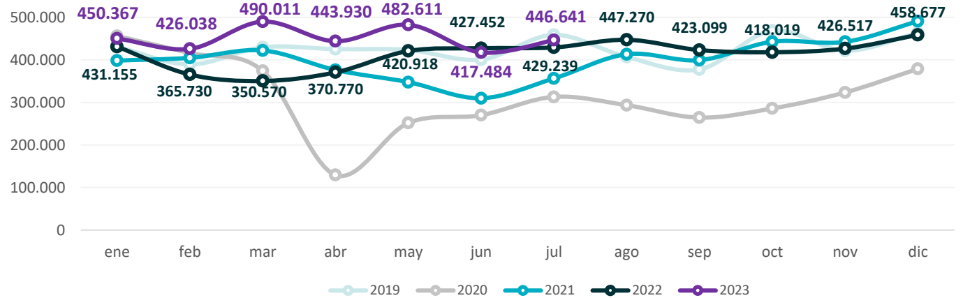
Gráfico 53. Provincia de Buenos Aires. Producción de nafta súper Período enero 2019 – julio 2023. En metros cúbicos
