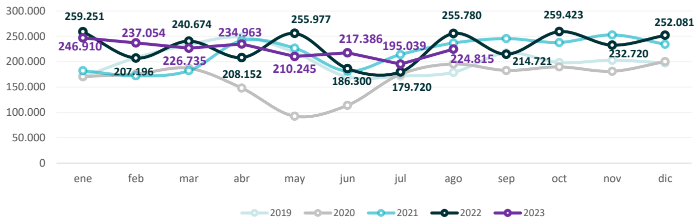
Gráfico 33. Provincia de Buenos Aires. Producción de hierro primario Período enero 2019 – agosto 2023. En toneladas
