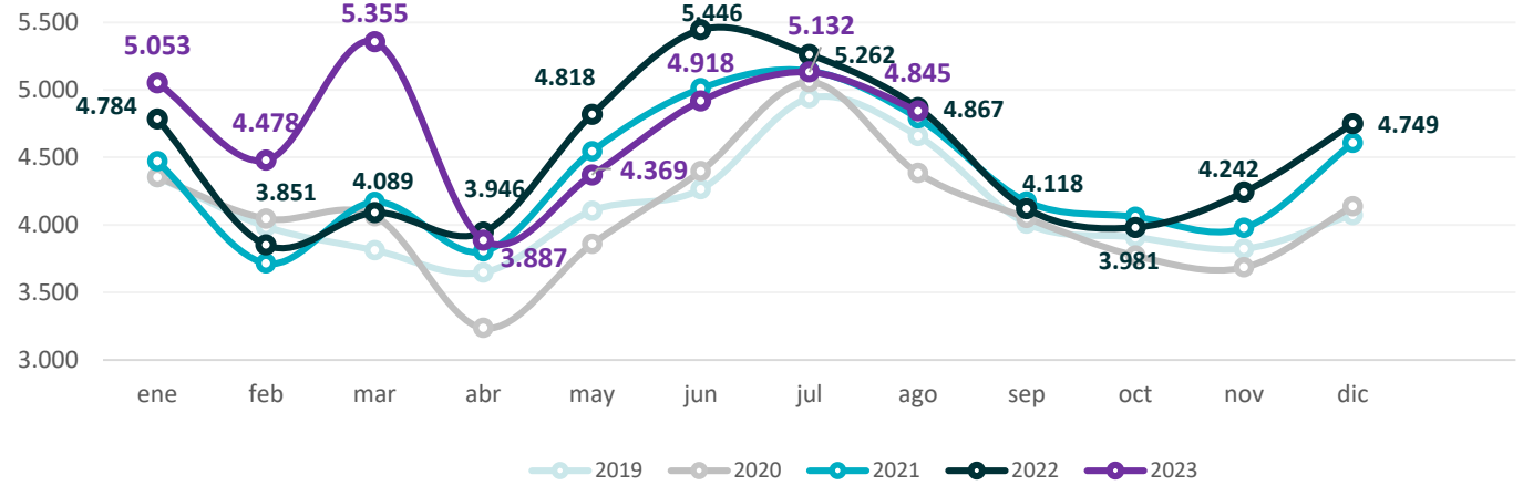
Gráfico 62. Provincia de Buenos Aires. Demanda eléctrica Período enero 2019 – agosto 2023. En Gwh
