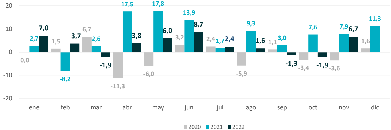
Gráfico 63. Provincia de Buenos Aires. Demanda eléctrica Período enero 2020 – octubre 2022. Variación porcentual interanual
