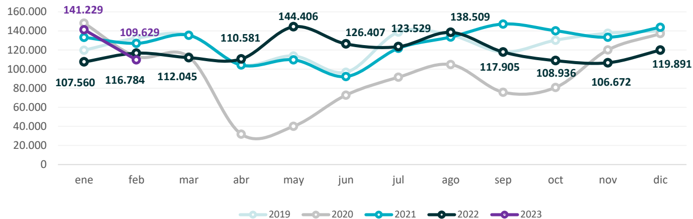
Gráfico 55. Provincia de Buenos Aires. Producción de nafta ultra Período enero 2019 – febrero 2023. En metros cúbicos
