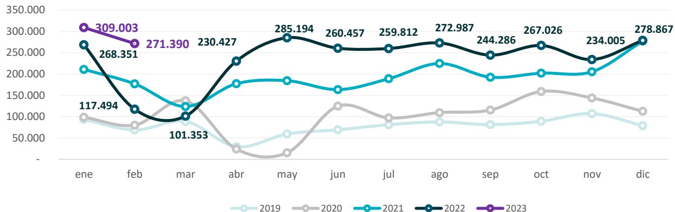
Gráfico 51. Provincia de Buenos Aires. Producción de gasoil ultra Período enero 2019 – febrero 2023. En metros cúbicos
